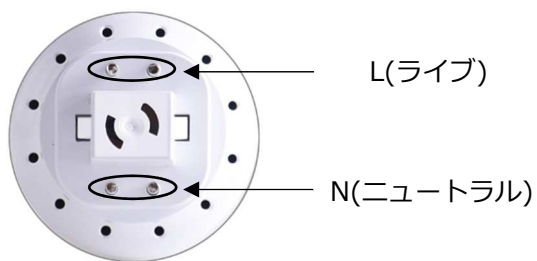
FHT 口金(GX24 p)
